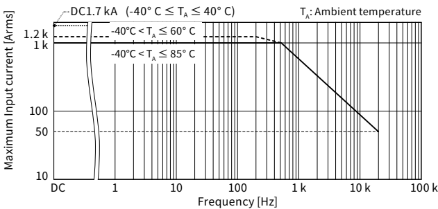
주파수특성 (대표특성 예)
